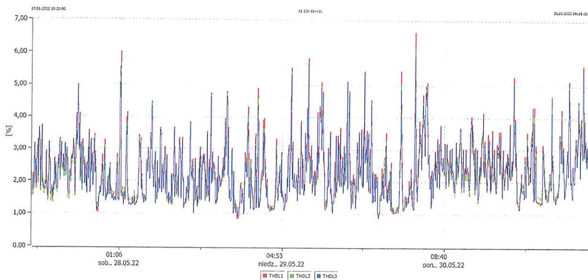
Wykres 3. THDU
