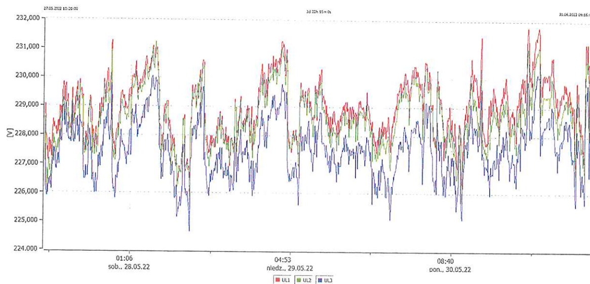
Wykres 1. Napięcie skuteczne średnie
