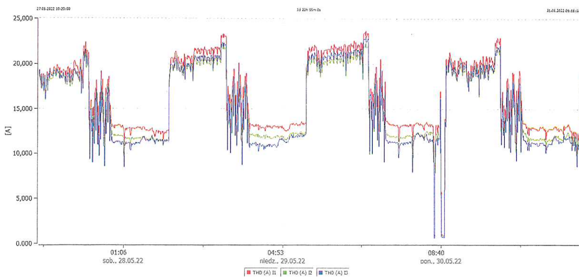
Wykres 4. THDI
