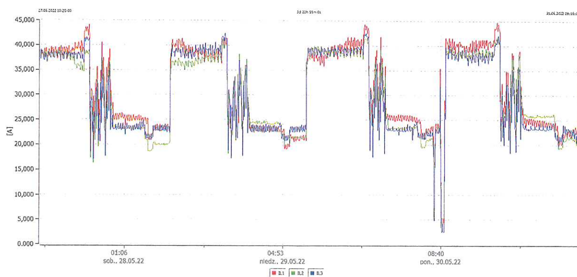
Wykres 2. Prądy skuteczne średnie
