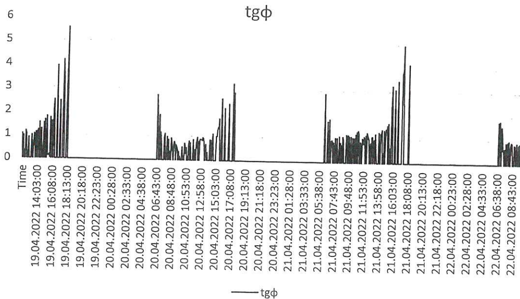
Wykres 9. Osiągany tg\phi
