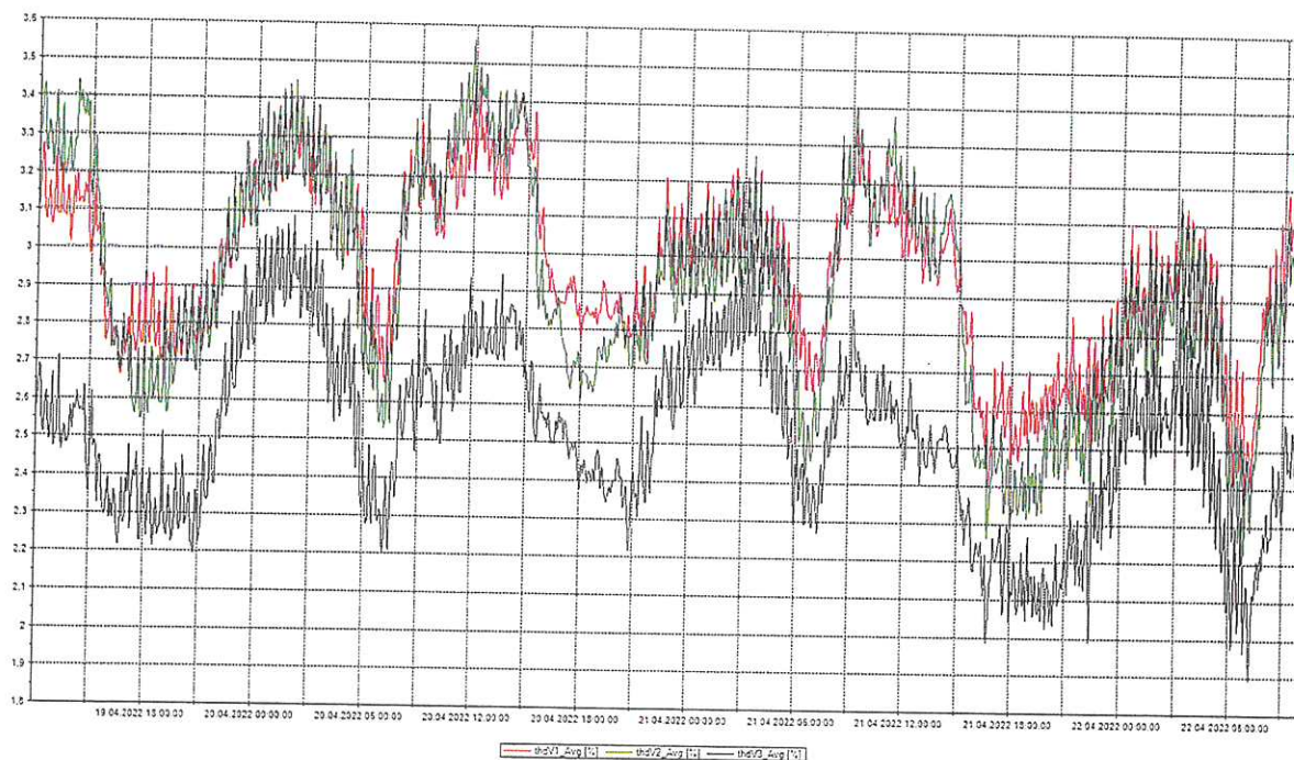
Wykres 3. THDU
