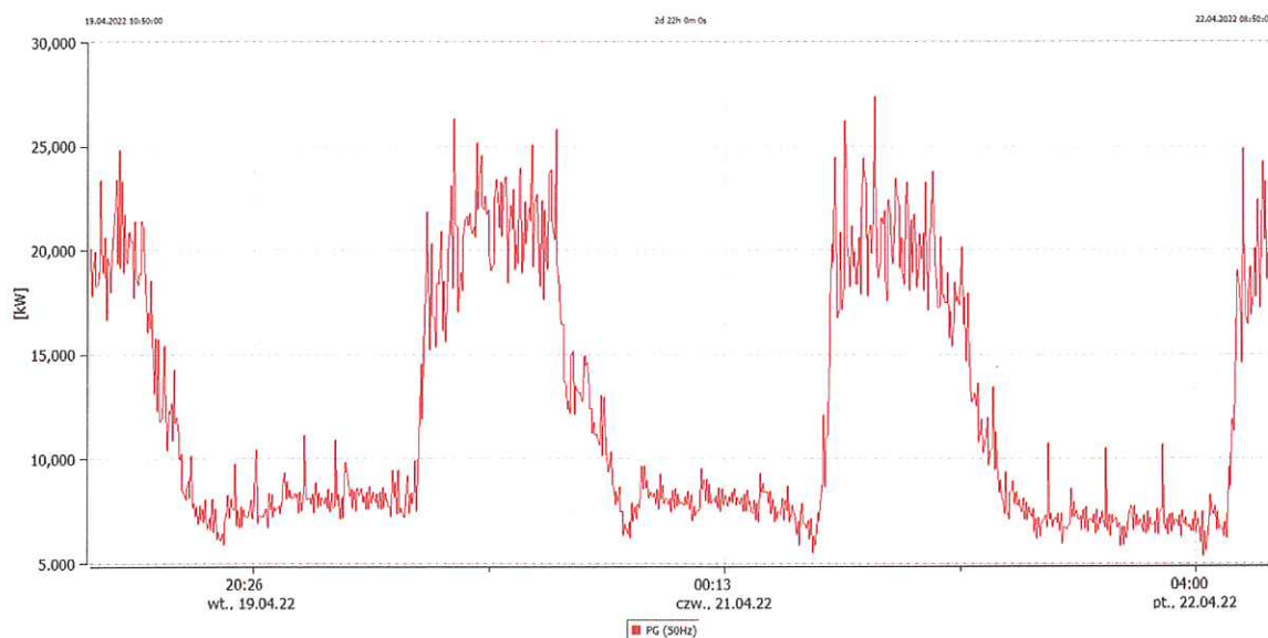
Wykres 5. Moc czynna
