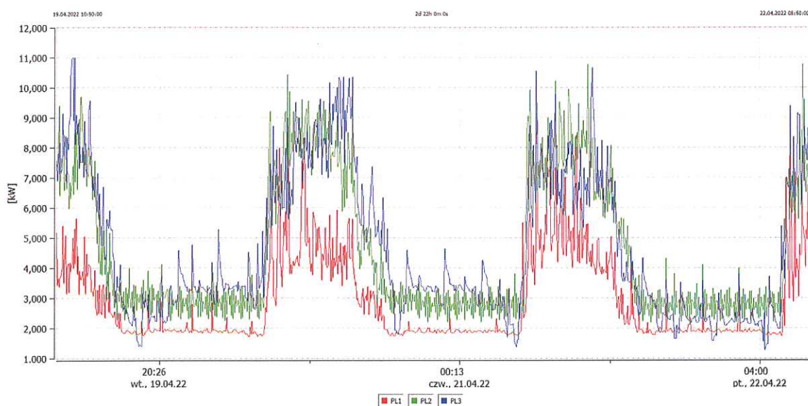
Wykres 6. Moc czynna w fazach
