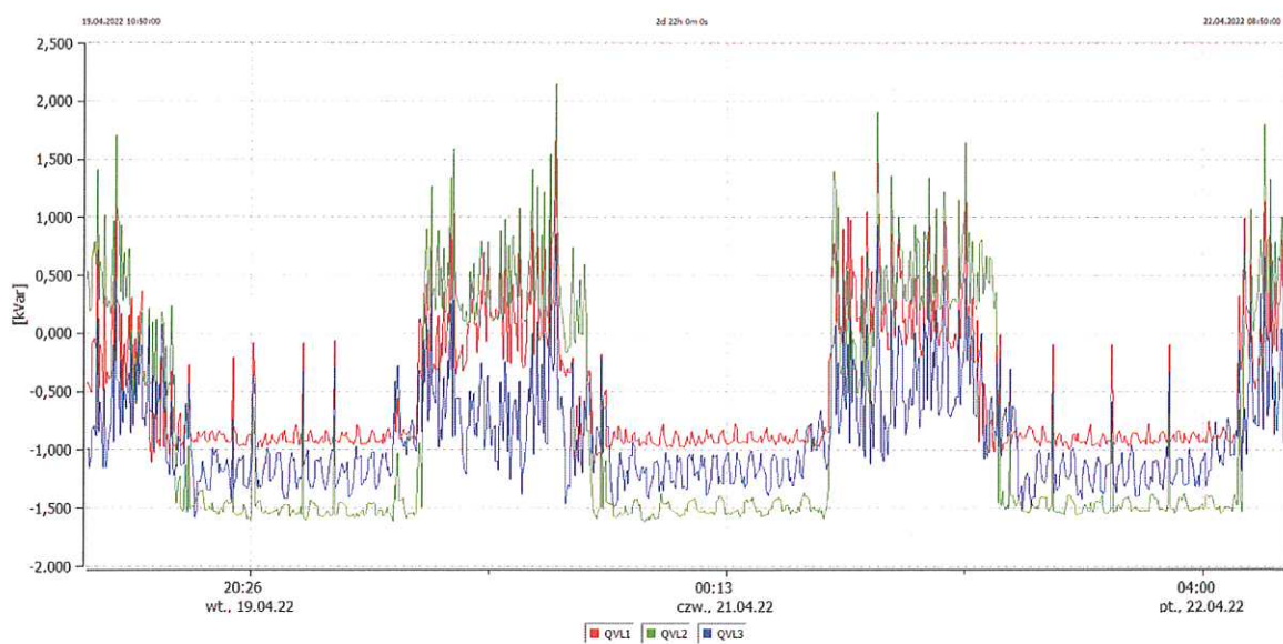
Wykres 8. Moc bierna w fazach
