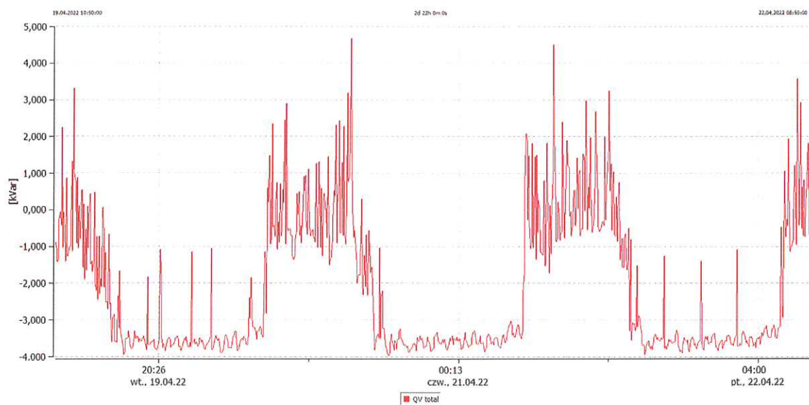
Wykres 7. Moc bierna
